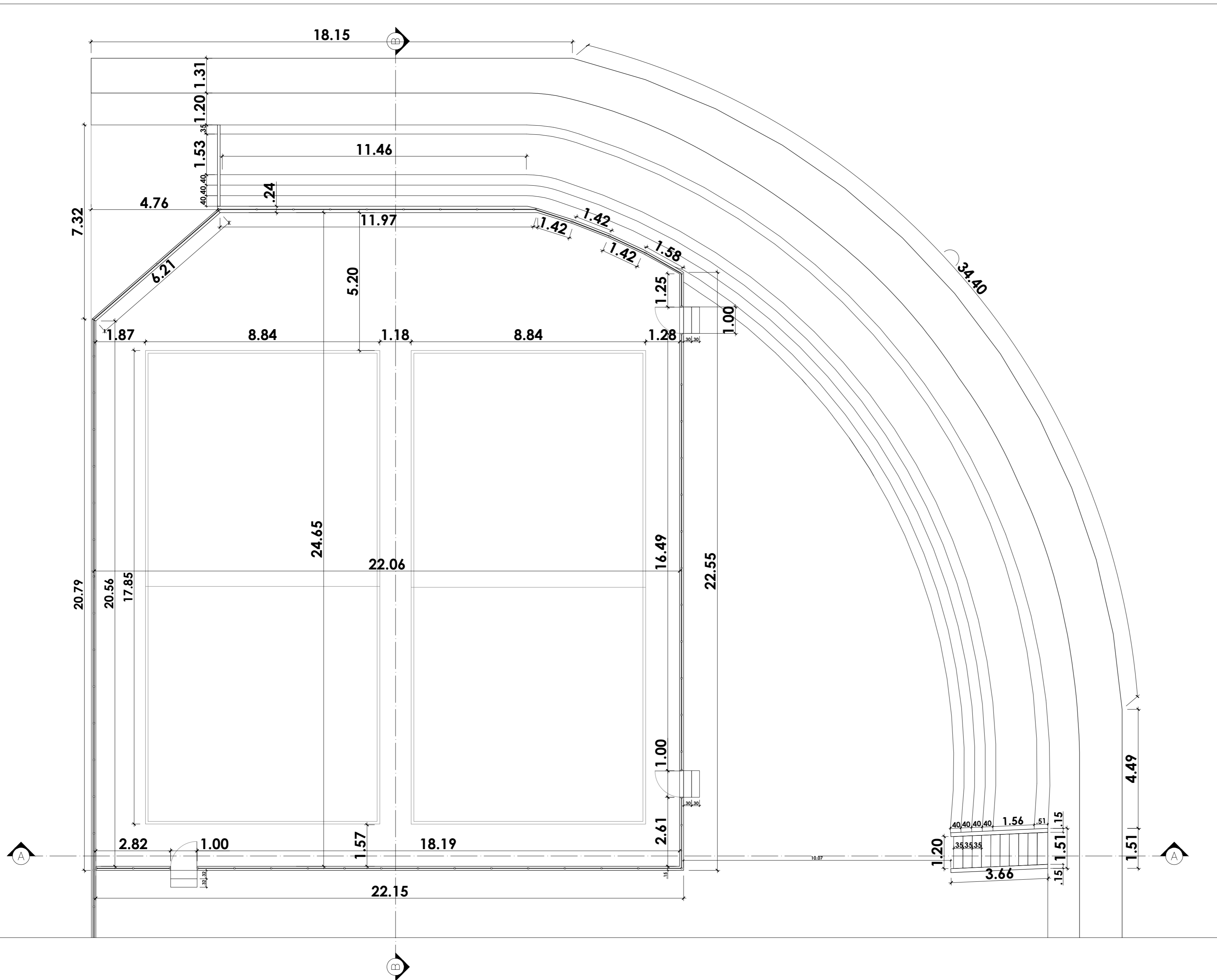
PLANTA BAIXA - COTADA ESC 1/100
