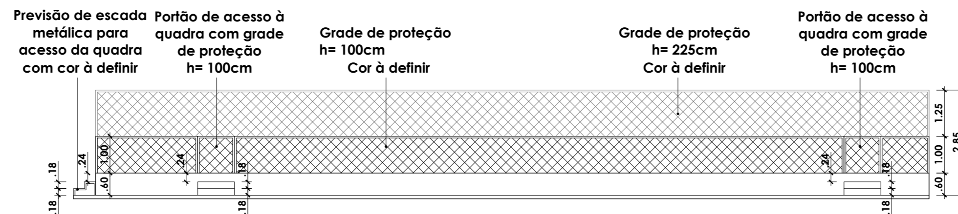
ELEVAÇÃO 02 ESC. 1/100
