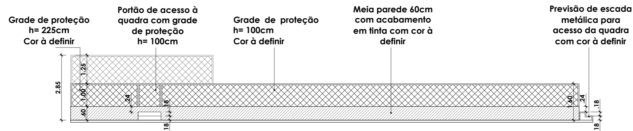
ELEVAÇÃO 01 ESC. 1/100
